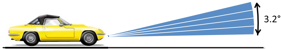
Abb. 4: Anordnung und vertikaler Sichtbereich des Automotive Laserscanners.
