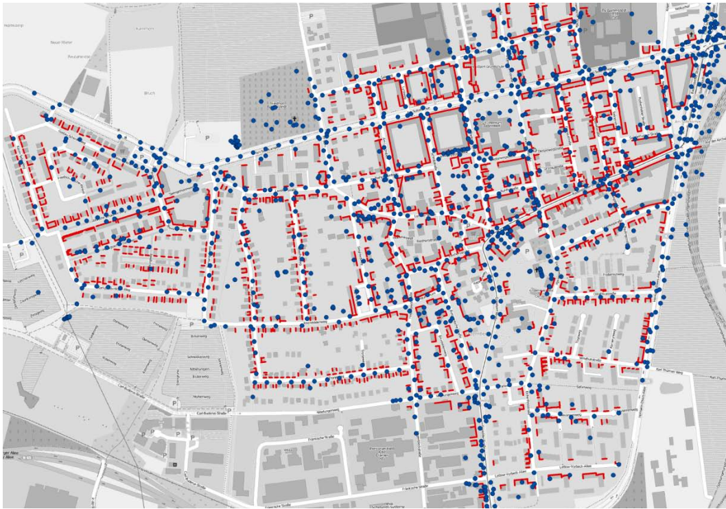
Abb. 1: Aus den Messungen des Mobile-Mapping-Systems extrahierte Stangen (blau) und Ebenen (rot). Hintergrundkarte: (OPENSTREETMAP, 2013).
