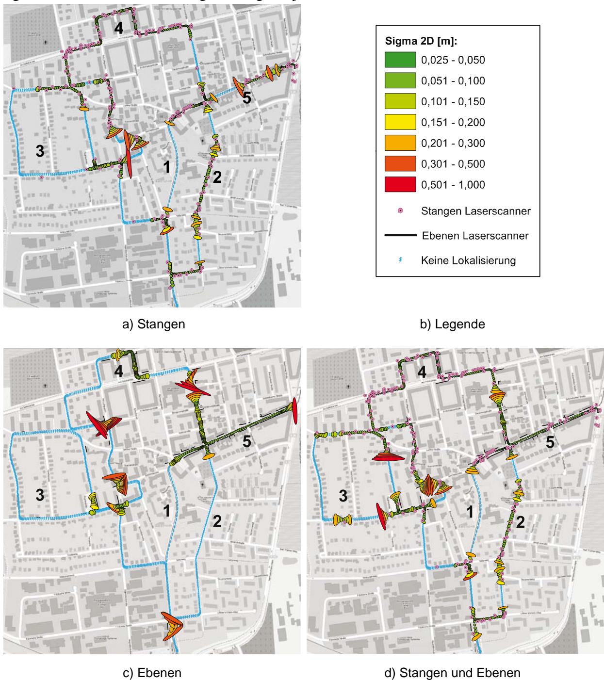
Abb. 7: Fehlerellipsen der Standpunkte im gewählten Testgebiet. Hintergrundkarte: (OPENSTREETMAP, 2013).
