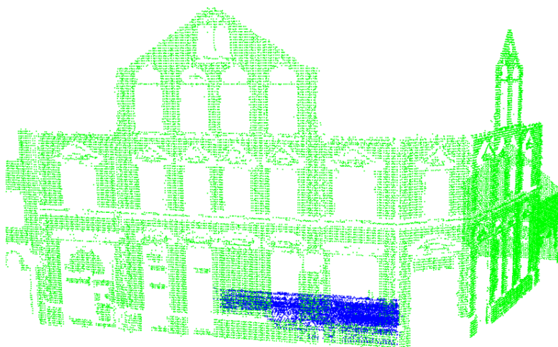
Abb. 5: Vergleich der vom Mobile Mapping System (grün) und vom Automotive-Laserscanner (blau) erfassten Punkte.
